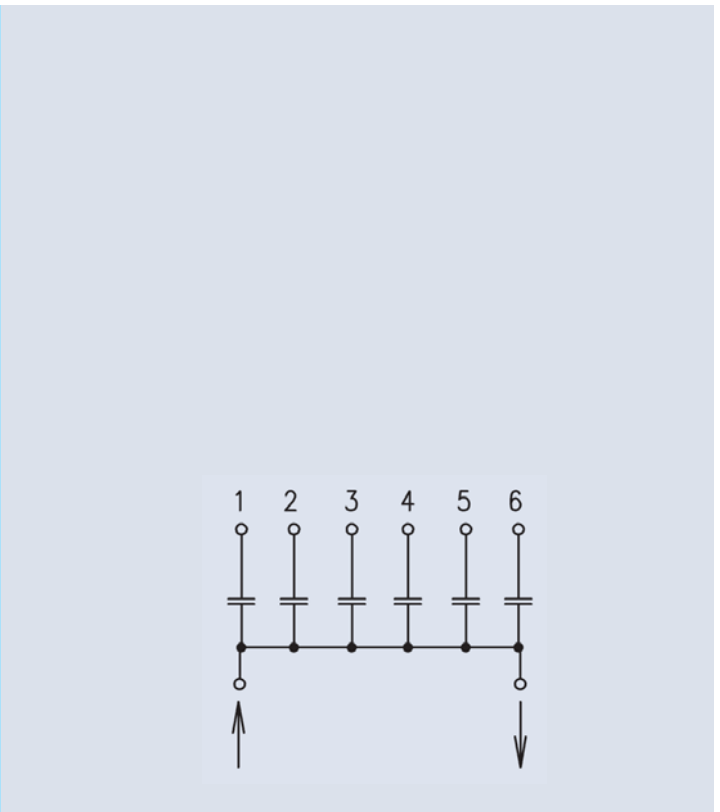
Diagram of connections / Диаграмма включения
