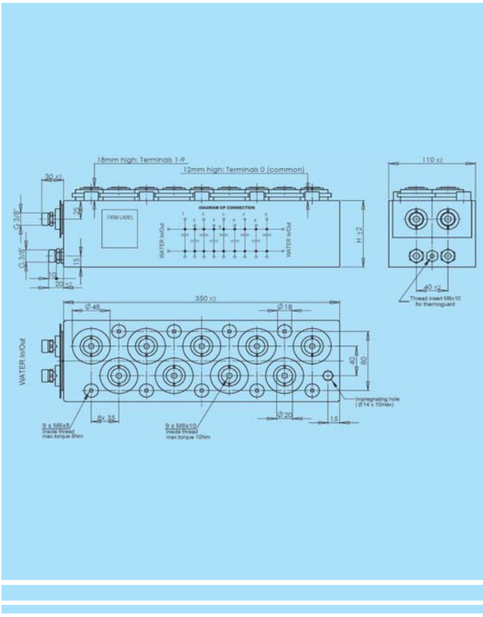
Dimensional Drawing 3 / Габаритный чертёж 3
