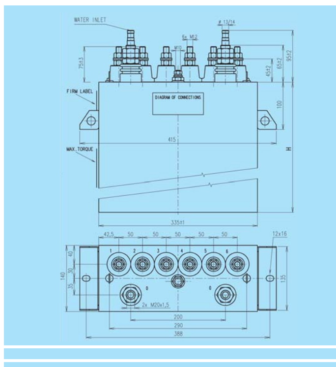
Dimensional Drawing 1 / Габаритный чертёж 1
