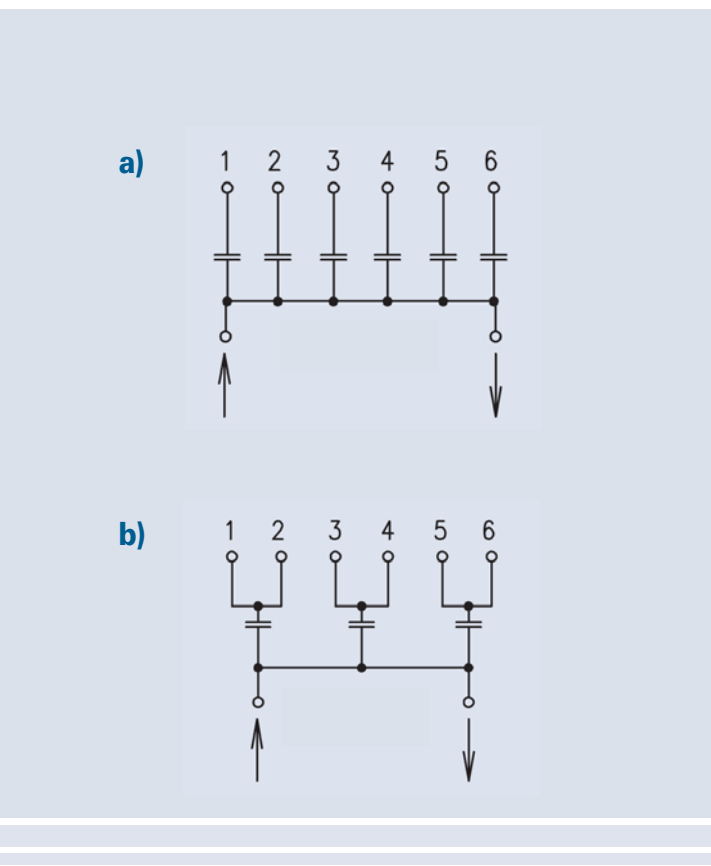
Diagram of connections / Диаграмма включения
