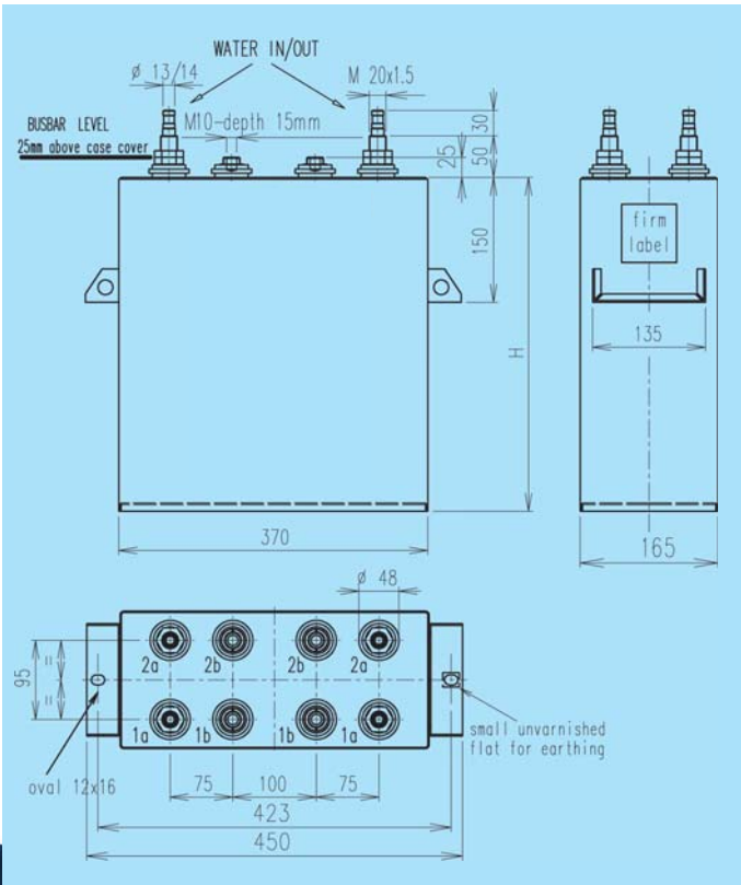
Dimensional Drawing 2 / Габаритный чертёж 2
