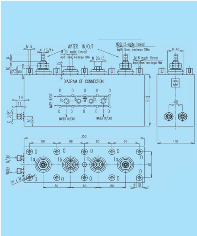
Dimensional Drawing 1 / Габаритный чертёж 1
